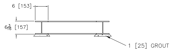
A-A
