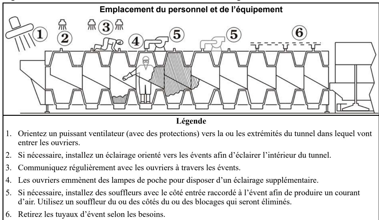
Figure 4. Sécurité dans le cadre de l'élimination des blocages du tunnel
