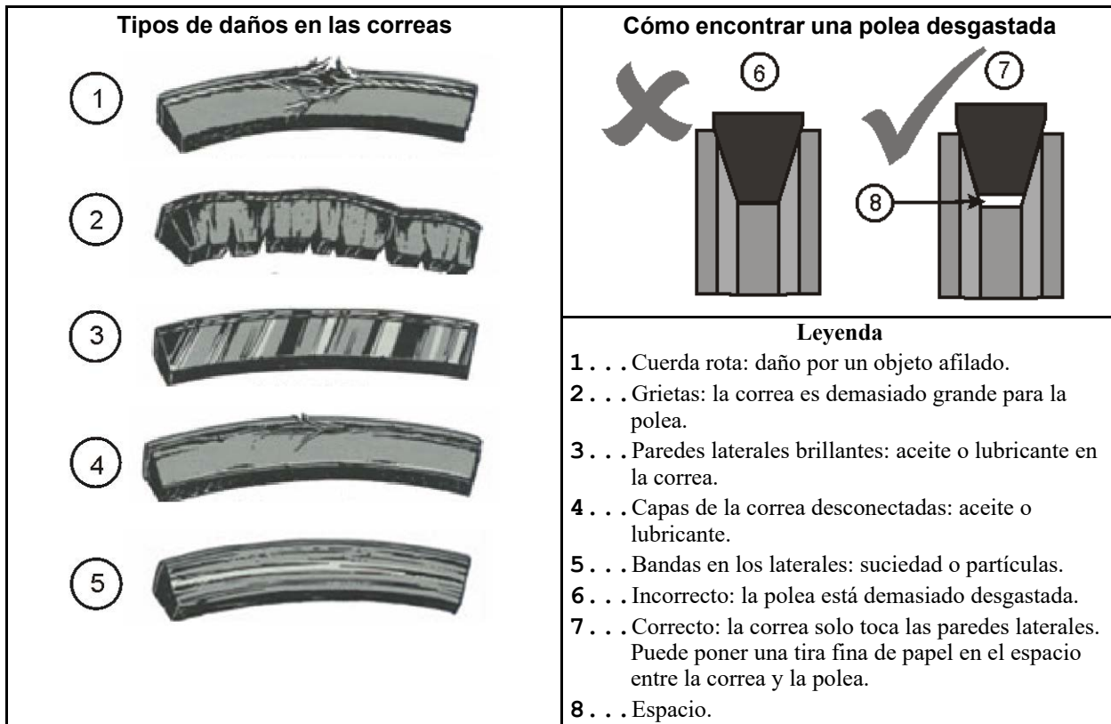
Ilustración 10. Condiciones a las que prestar atención de las correas y las poleas
