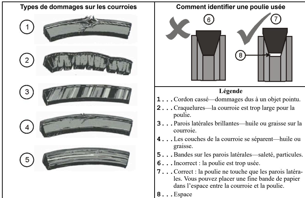
Figure 10. Conditions des courroies et des poulies à contrôler
