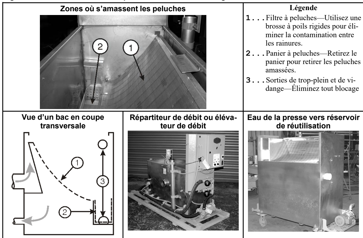
Figure 28. Réservoir PulseFlow®—Tunnels de lavage PulseFlow® CBW
