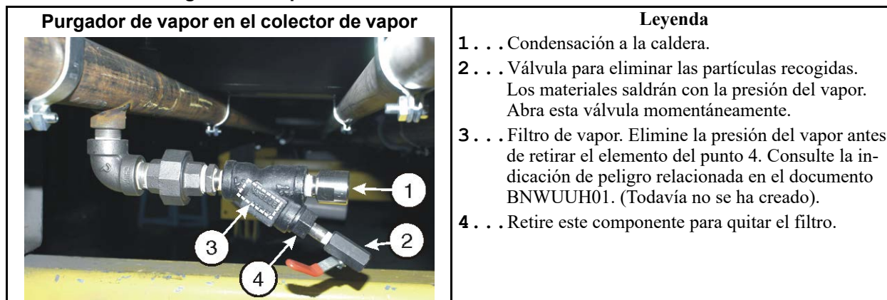
Ilustración 31. Purgador de vapor
