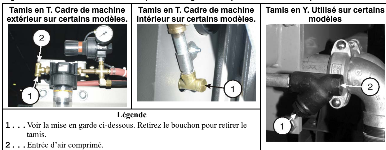
Figure 17. Tamis d'entrée d'air comprimé. Il s'agit d'exemples. Votre machine peut être différente.
