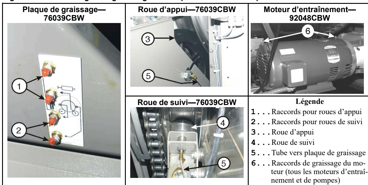
Figure 23. Points de graissage. Il s'agit d'exemples. Votre machine peut être différente.
