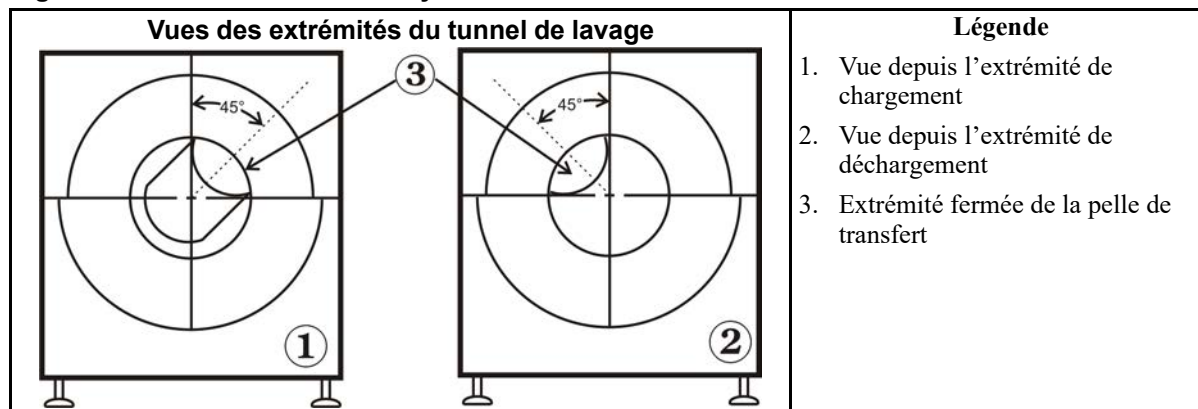
Figure 2. Positionnement des cylindres
