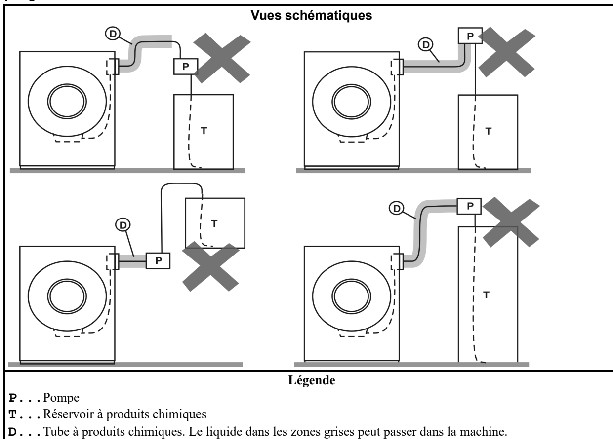
Figure 6. Configurations incorrectes qui laissent les produits chimiques passer dans la machine par gravité
