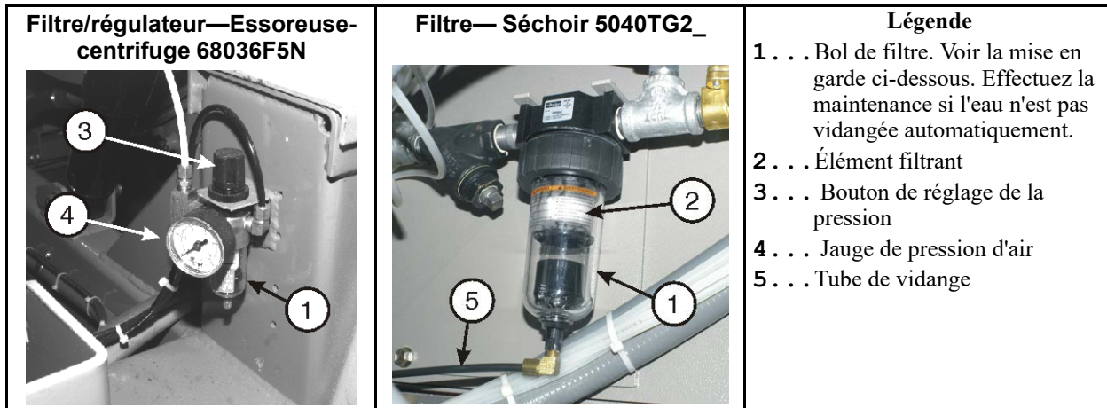
Figure 18. Filtre de conduite d'air à purge automatique servant à supprimer l'humidité et d'autres contaminations. Il s'agit d'exemples. Votre machine peut être différente.
