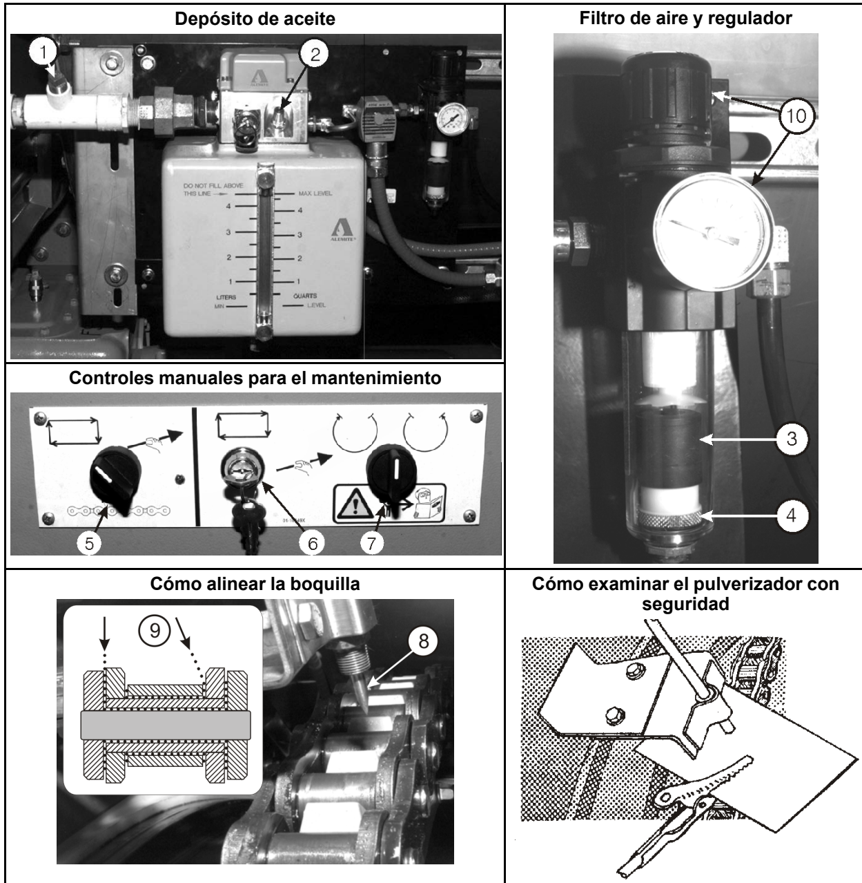
Ilustración 25. Sistema de nebulización de aceite para la cadena de transmisión
