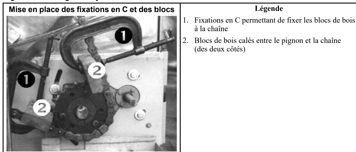
Figure 3. Blocage des cylindres
