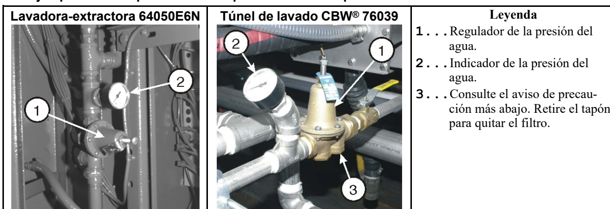
Ilustración 15. Regulador de la presión del agua para la descarga de productos químicos. Estos son ejemplos. Su máquina de lavado puede tener un aspecto diferente.
