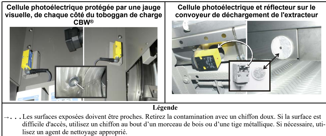
Figure 21. Détecteurs de proximité Ce sont des exemples. Votre machine peut être différente.
