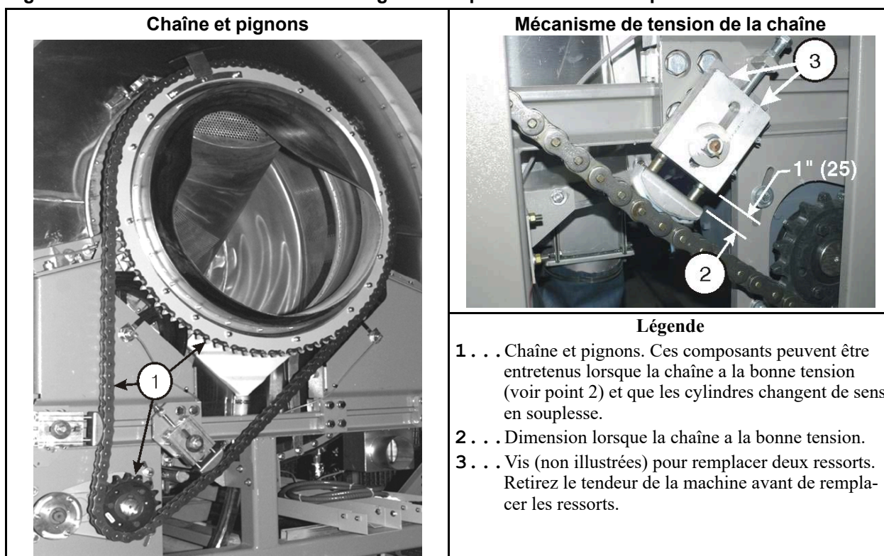
Figure 26. Chaîne de transmission. Il s'agit d'exemples. Votre machine peut être différente.
