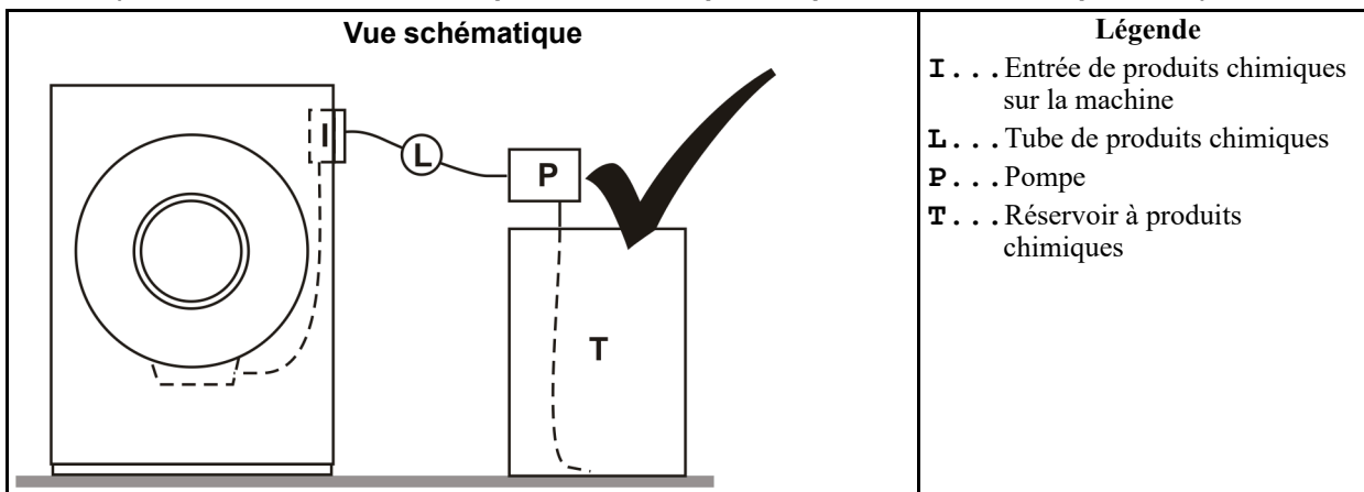
Figure 8. Une configuration qui empêche l'écoulement dans la machine lorsque la pompe est arrêtée (si le réservoir et le tube de produits chimiques ne présentent aucune pression)
