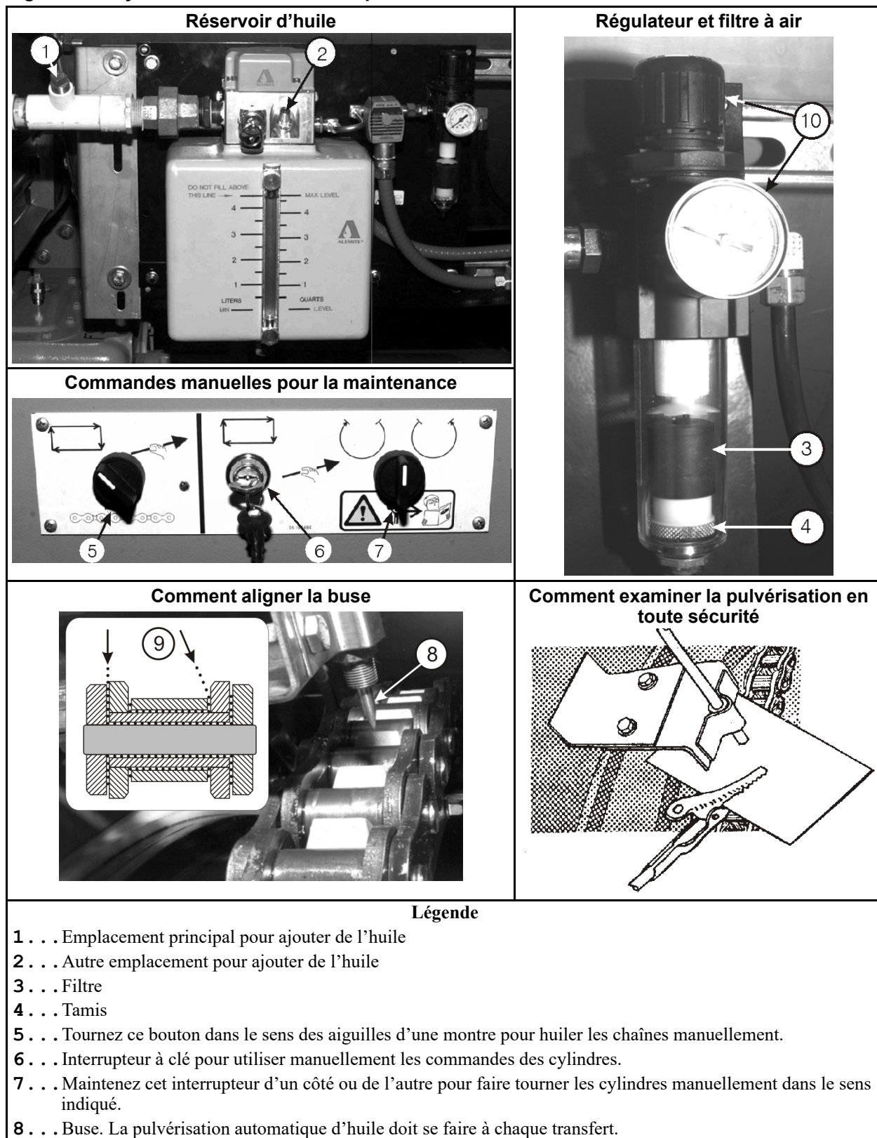
Figure 25. Système à brouillard d'huile pour la chaîne de transmission
