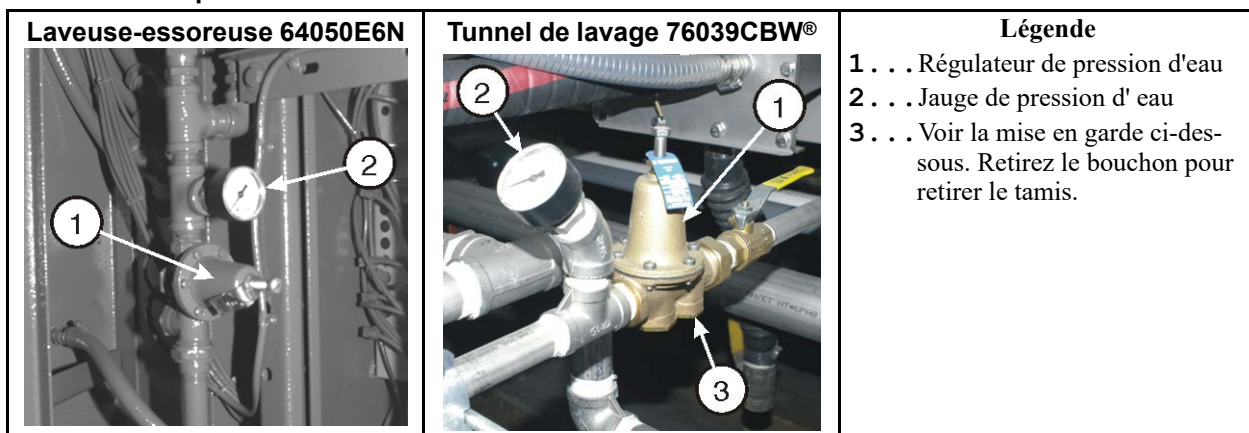
Figure 15. Régulateur de pression d'eau de rinçage des produits chimiques. Il s'agit d'exemples. Votre machine peut être différente.
