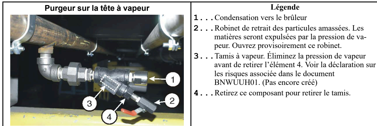
Figure 31. Purgeur
