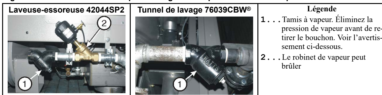
Figure 16. Tamis d'entrée de vapeur. Il s'agit d'exemples. Votre machine peut être différente.
