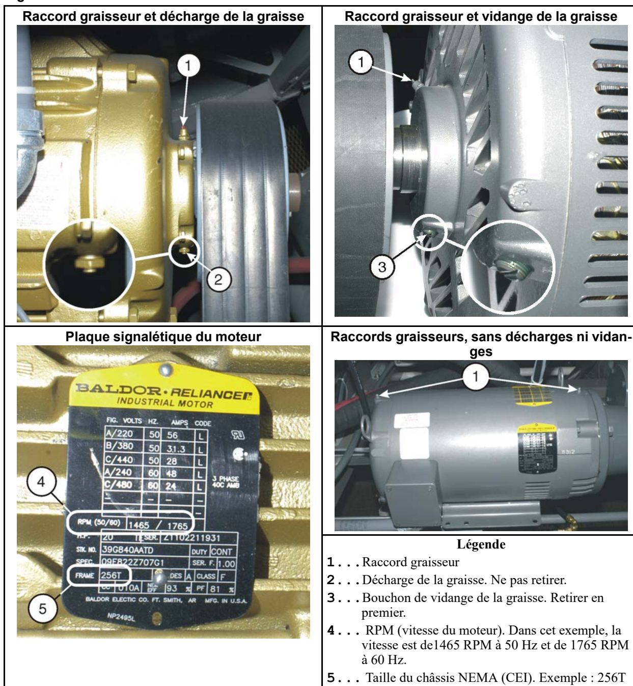
Figure 9. Conditions de lubrification du moteur
