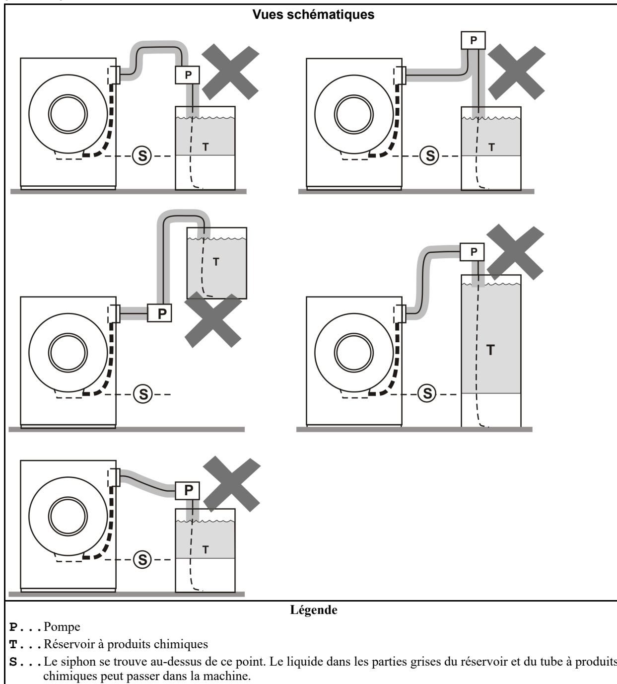
Figure 5. Configurations incorrectes qui laissent les produits chimiques passer dans la machine par un siphon
