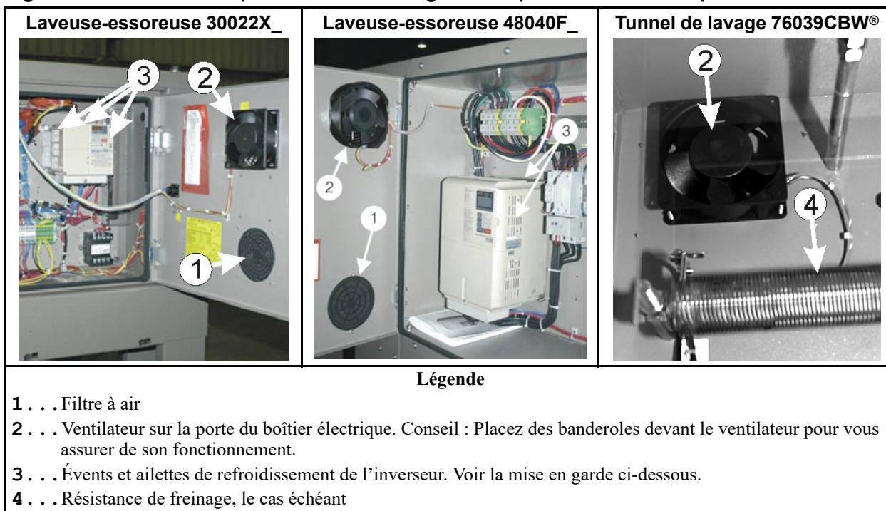
Figure 12. Boîtier électrique et inverseur Il s'agit d'exemples. Votre machine peut être différente.
