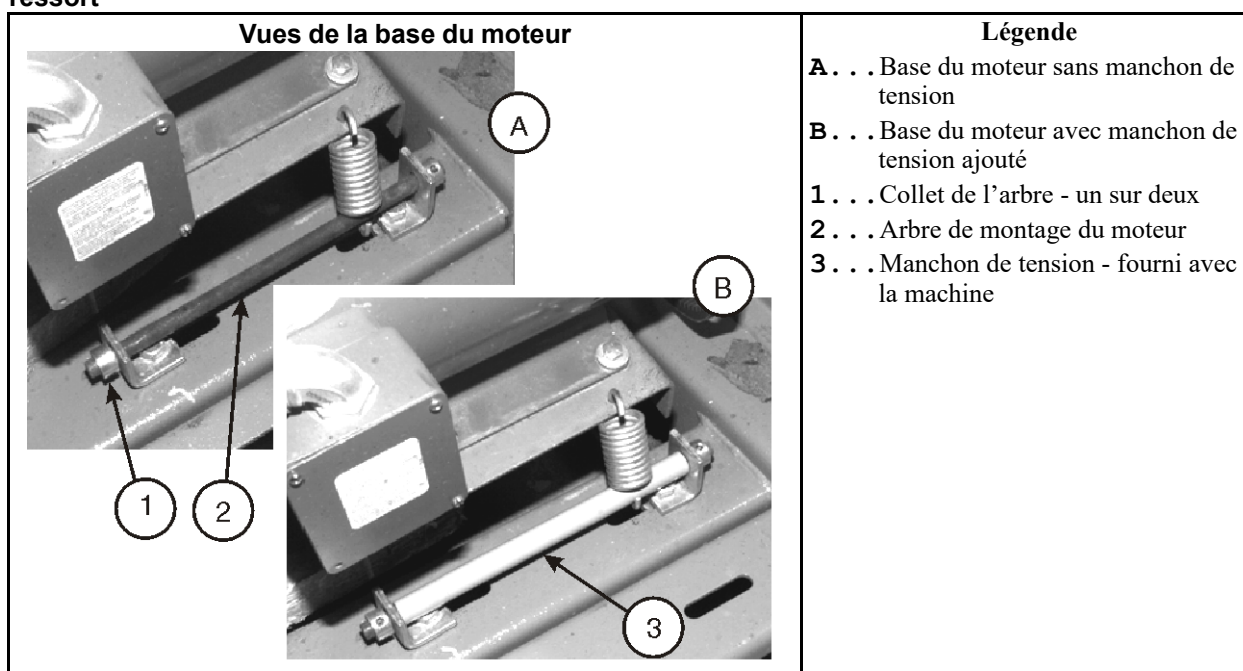
Figure 11. Comment régler la tension de la courroie sur une machine qui utilise la tension du ressort
