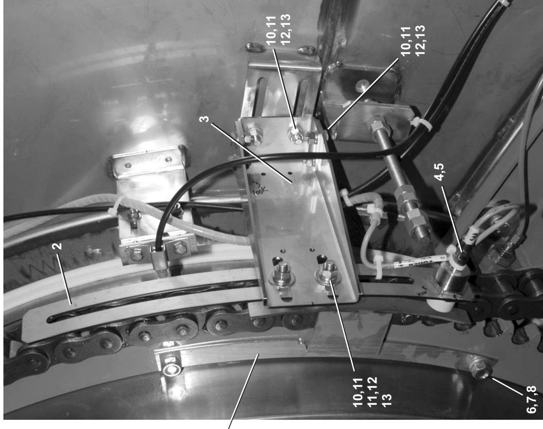
Counter Clockwise Limit Switch (D)
